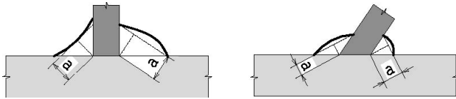
Fig. 4.2.6 - Definizione dell'area di gola per le saldature a cordone d'angolo
