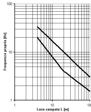
Fig. 5.2.7 - Limite delle frequenze proprie n_0 in Hz in funzione della luce della campata
