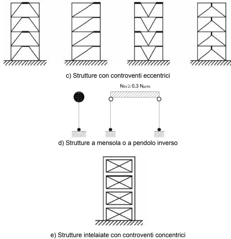
Fig. 7.5.1. - Tipologie strutturali
