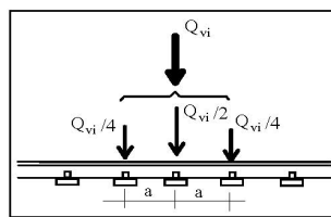
Fig. 5.2.3 - Distribuzione longitudinale dei carichi assiali
